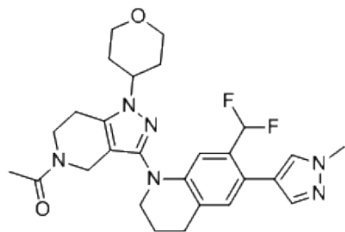
PC-6164101, DMSO-d6
